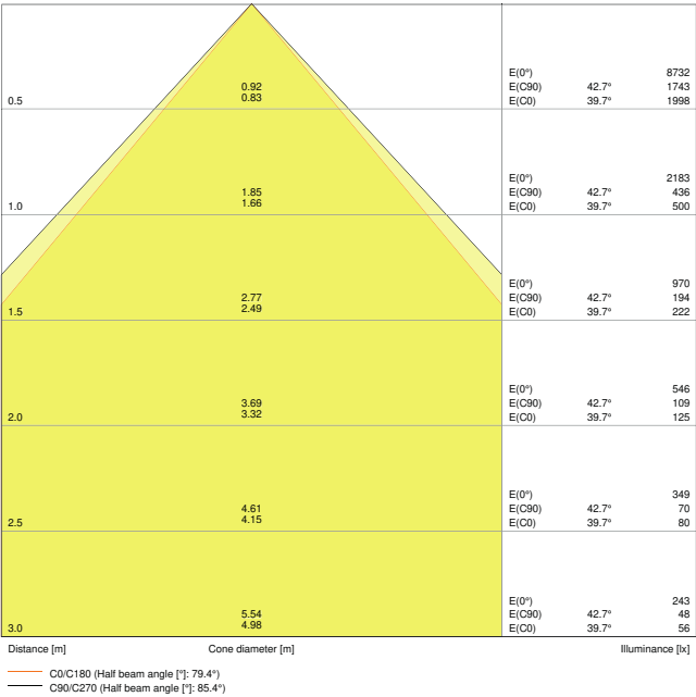
PL PFM 625 DALI 36W 3000K UGR19 LDT
