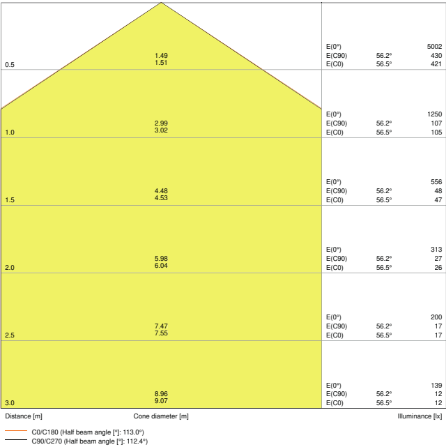
PL PFM 625 30W 4000K LDT
